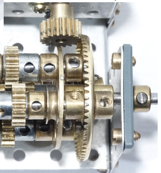
Planetenpaar
